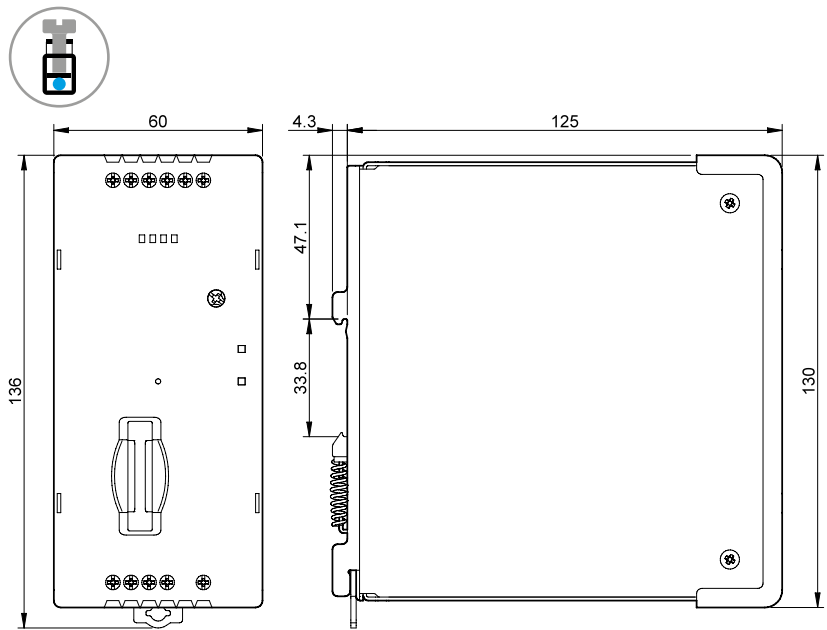
Type 78.2E Box clamp
