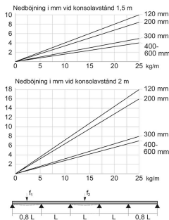
Diagrammet gäller för ett innerfack f i - d v s alla fack utom de två yttersta. För att få samma lastbärande yterfack f 1 ska konsolavståndet vara 80 % av ett innerfack.
