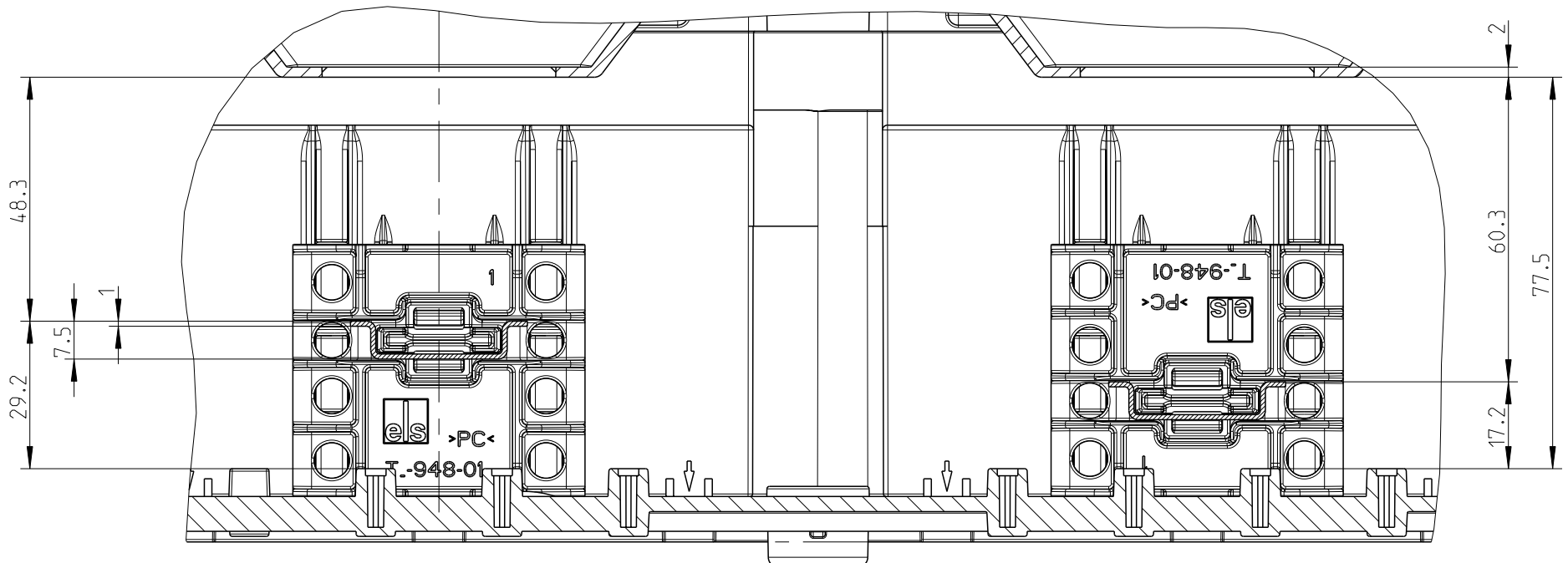
A-A 4:5 Detail um 90° gedreht
